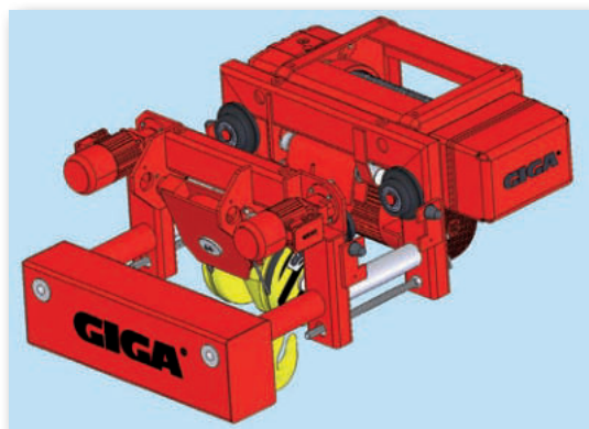
Электрический канатный тельфер с укороченной строительной высотой, грузоподъёмность 10т, тун GHM 10000-20-4/1-6M,Z
