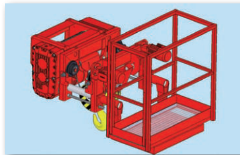
Тельфер GIM 12500 с сервисной «корзиной»
