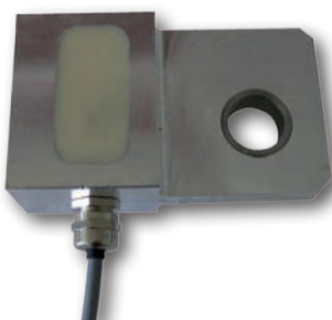
Тензометр для тельфера серии GHM, устанавливается в жѐстком захвате каната тельфера
